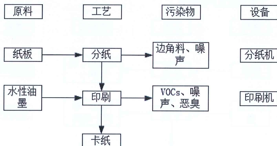
图 2-2 卡纸生产工艺流程及产污环节示意图
