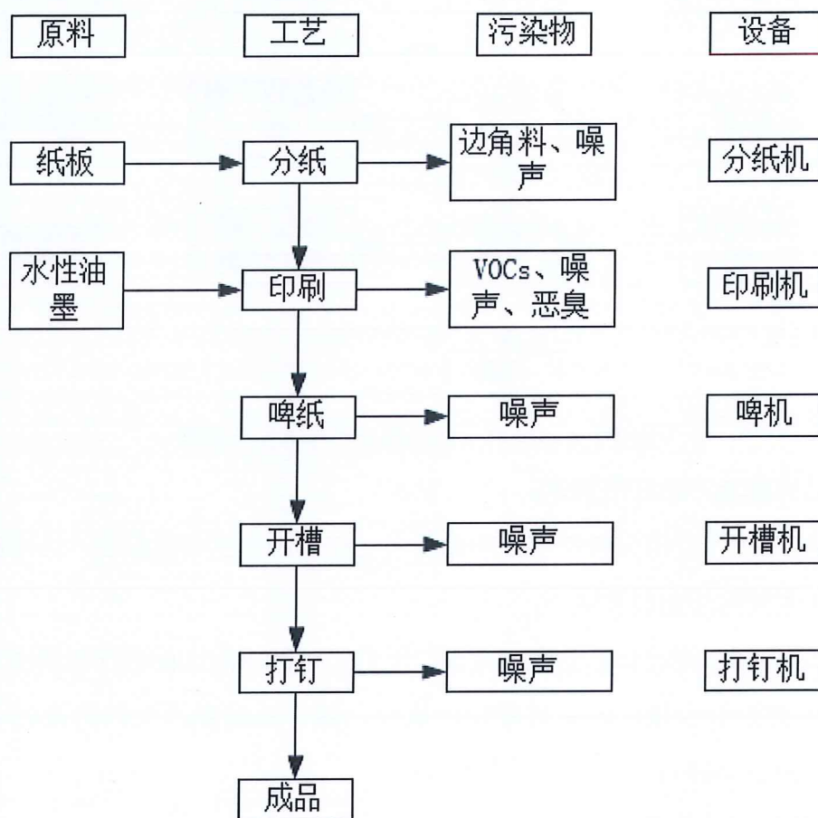
图 2-1 纸箱生产工艺流程及产污环节示意图
